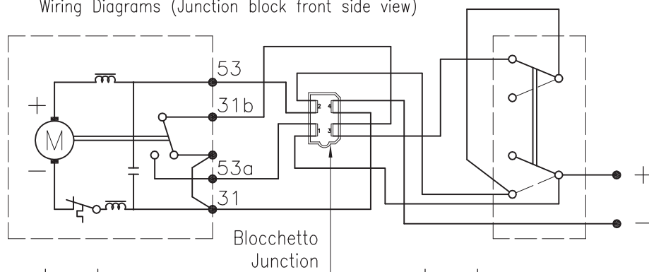
Schema di connessione (Blocchetto visto di fronte) Wiring Diagrams (Junction block front side view)
